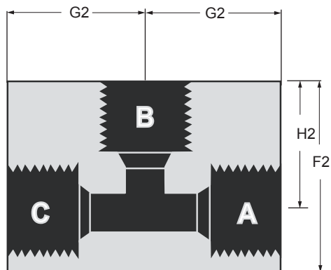
Тройник
