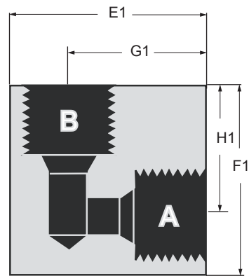
Уголок
